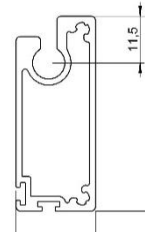
Alaprofiil: L19,5 x K48mm
