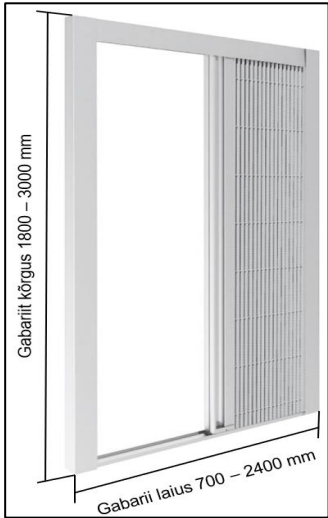
Voldik putukavõrk (must) Tõmbeprofiil liigub rullikuga alaprofiilil
